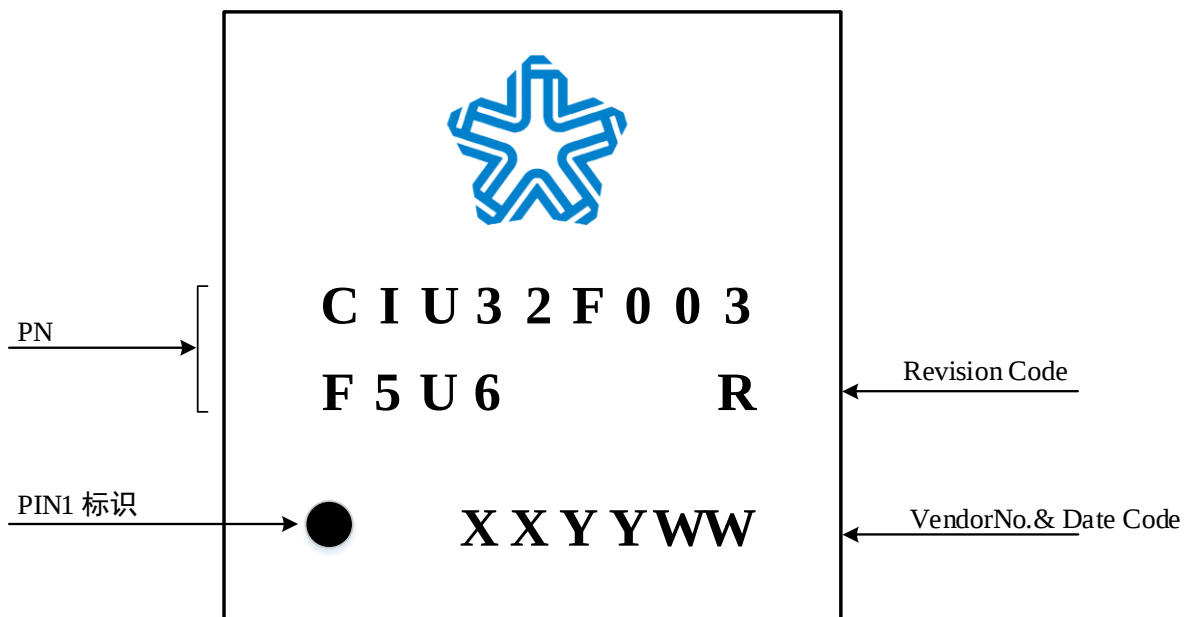
图 5-7 QFN20 封装丝印信息说明
